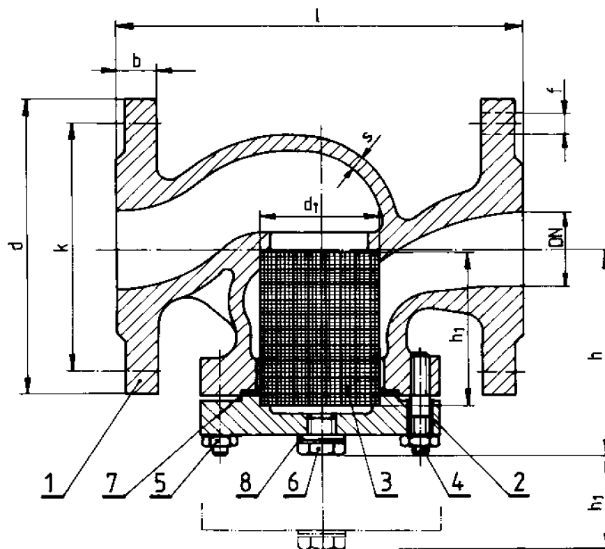
PRIMJER OZNAČAVANJA FILTRA IZVEDBE B, NAZIVNOG PROMJERA DN 150 : FILTAR SB 11256-B 150
